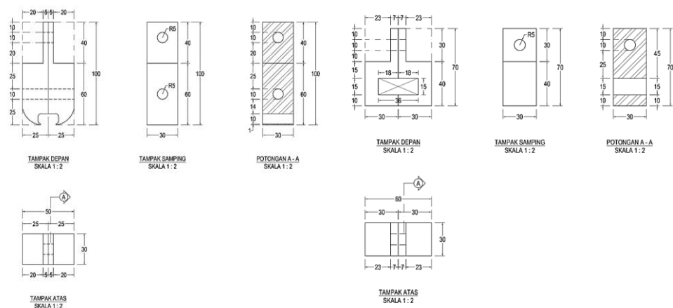
Gambar 3. Desain Penjepit Penambat E-Clip dan DE-Clip
