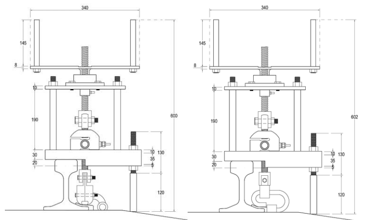
Gambar 2. Desain 2 Dimensi Alat Generasi Kedua
