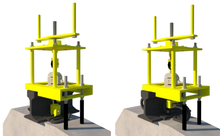
Gambar 4. Tampilan 3 Dimensi Alat Generasi Kedua
