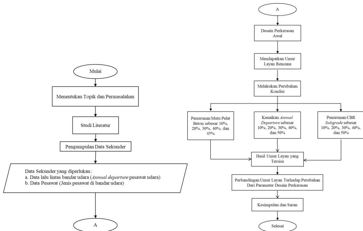
Gambar 2. Bagan Alir Rencana Kerja
