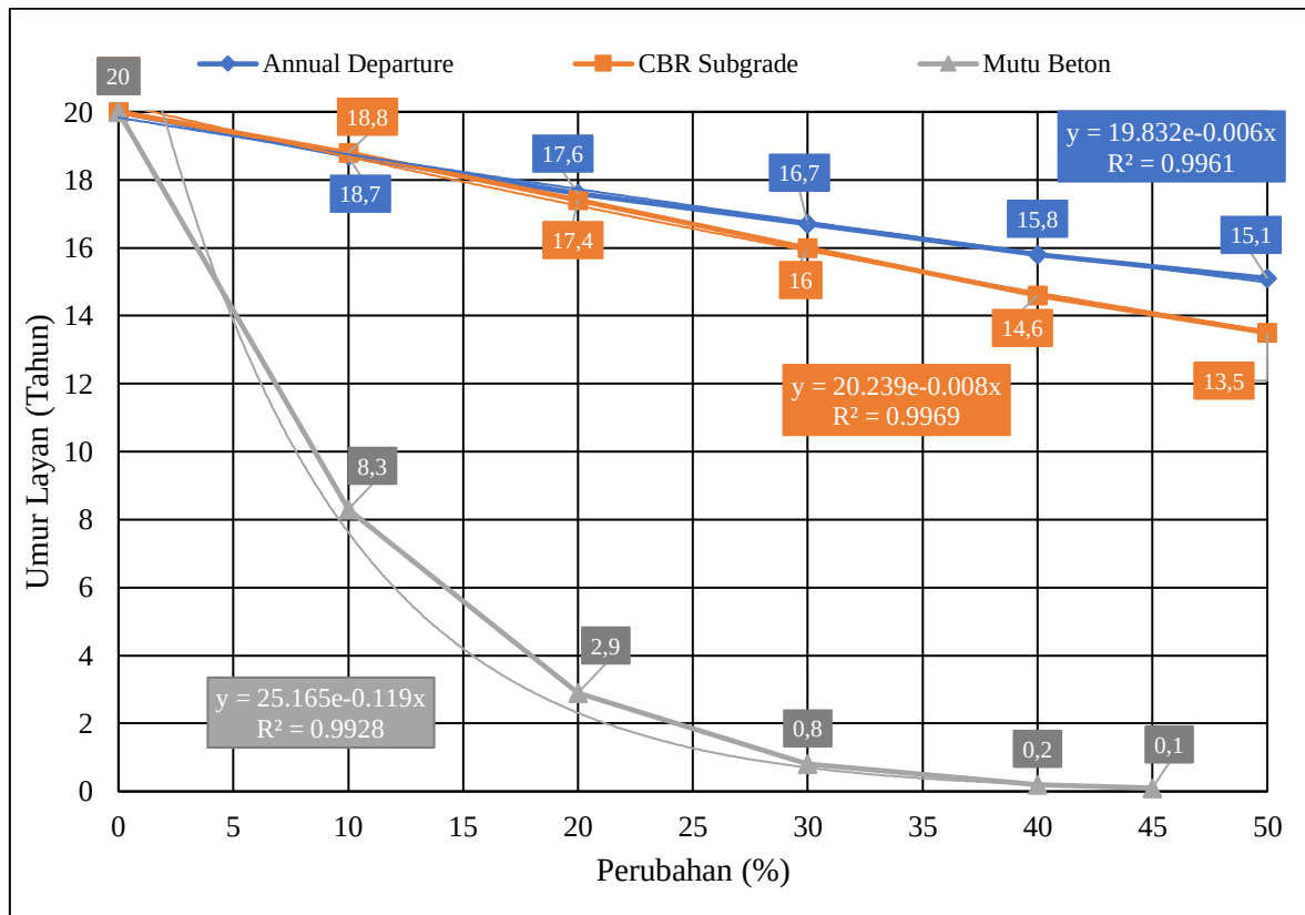
Gambar 3. Grafik Sisa Umur Layan Terhadap Perubahan Annual Departure , CBR Subgrade dan Mutu Beton
