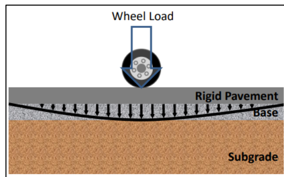
Gambar 1. Ilustrasi Pembebanan Perkerasan Kaku
