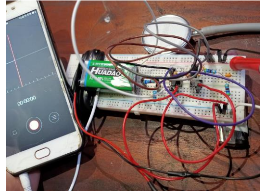
Gambar 4. Stetoskop modifikasi yang terhubung dengan perekam suara
